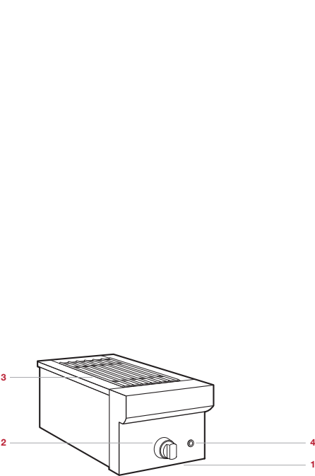
Módulo para exterior (se muestra el módulo con quemador).
