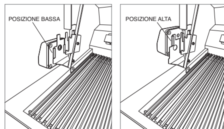
Posizione girarrosto in basso.
