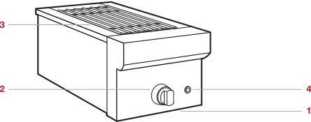
户外燃气烤架（所示为燃烧器模块）。
