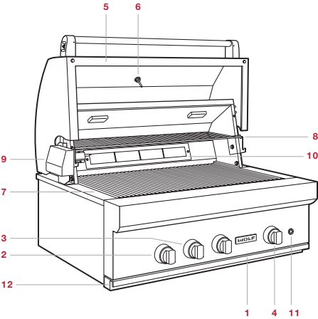
Outdoor-Gasgrill (Modell ICBOG36 abgebildet)
