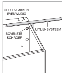
Breng de achterkant van de versterking op gelijke hoogte.
