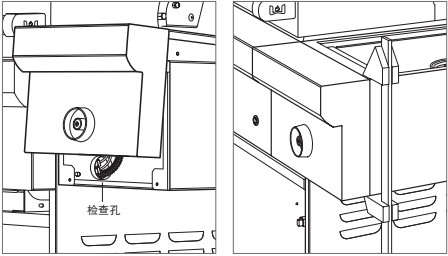
定位侧壁燃烧器。
