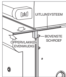
Breng de voorkant van de versterking op gelijke hoogte.
