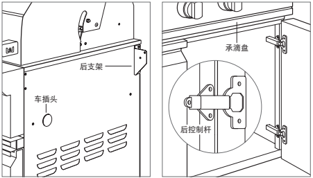
卸下后支架和插头。
