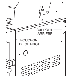
Retirez le support arrière et le bouchon.
