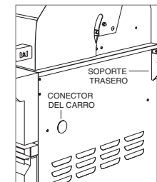
Retire el conector y el soporte trasero.
