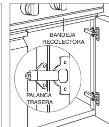
Retire la puerta del carro.
