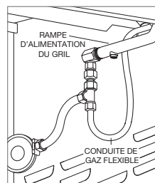
Raccordement au propane (LP).
