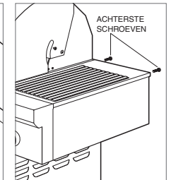
Bevestig de zijbrander.
