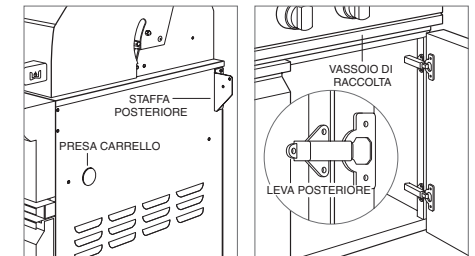
Rimuovere la staffa posteriore e la presa.
