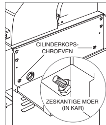
Bevestig de versterking.
