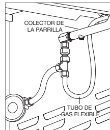
Conexión de gas LP.
