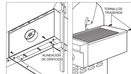
Alineación del orificio.
