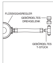
Flüssiggasregler-Baugruppe
