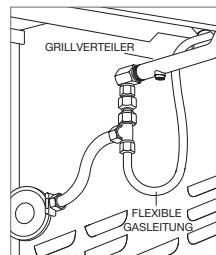
Flüssiggasanschluss
