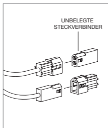
Steckverbinder
