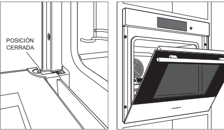
Pestillo de la bisagra de la puerta del horno Puerta abierta a 30°
