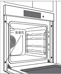
烤箱安装
