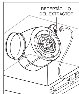
Conexión del extractor
