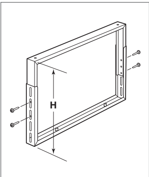
Ajuste de los soportes
