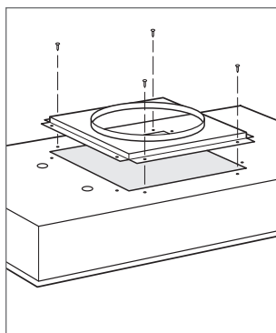
Instalación de la brida
