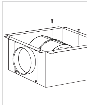
Installation du ventilateur interne
