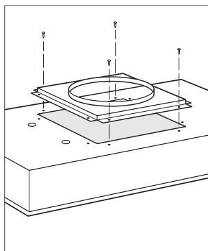
Installation de la bride
