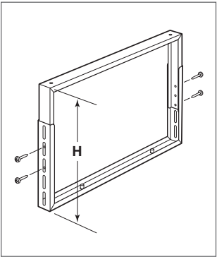
Réglage des supports
