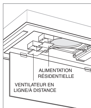
Connexions
