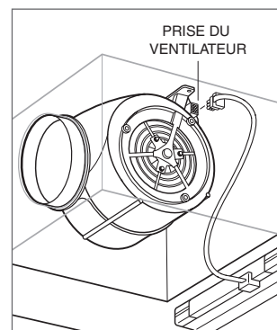
Connexion du ventilateur
